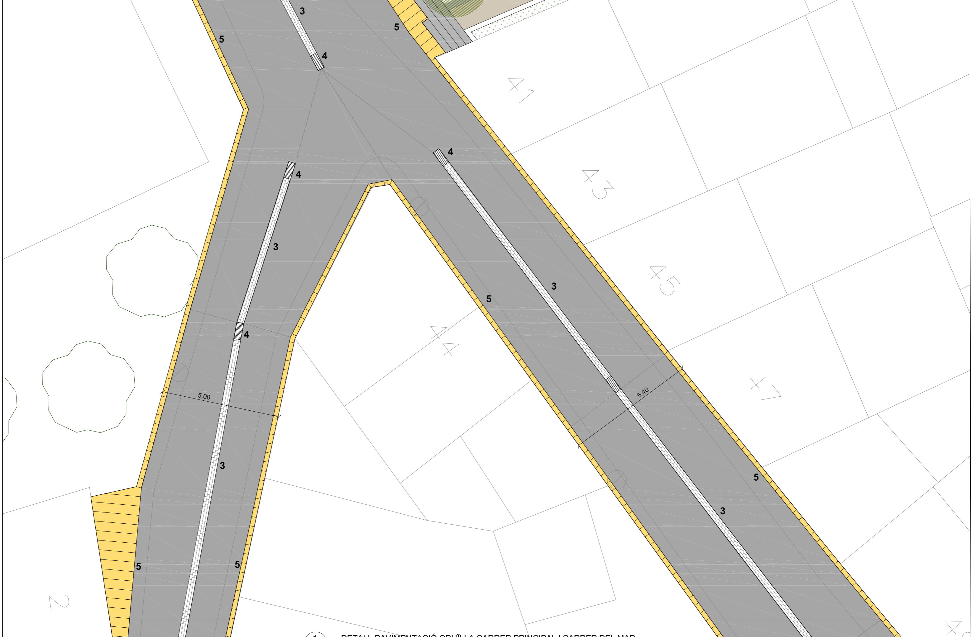
1 0.4 DETALL PAVIMENTACIÓ CRUÏLLA CARRER PRINCIPAL I CARRER DEL MAR E: 1/100
